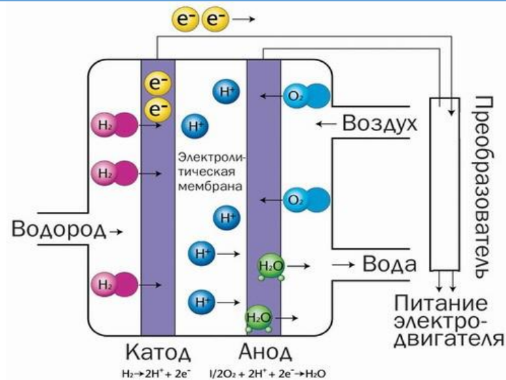
Рис. 3. Принципиальная схема топливного элемента.
